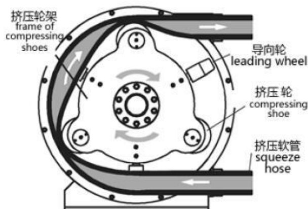
泵体结构原理
