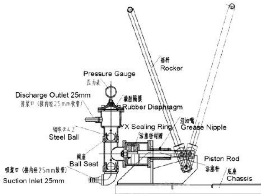
结构图 Structure Drawing
